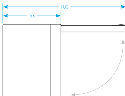
Розетка IP20
