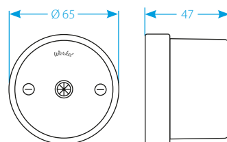
TV-розетка
